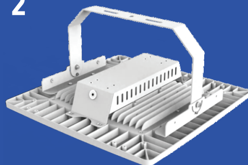
Montaža sa nosačem
